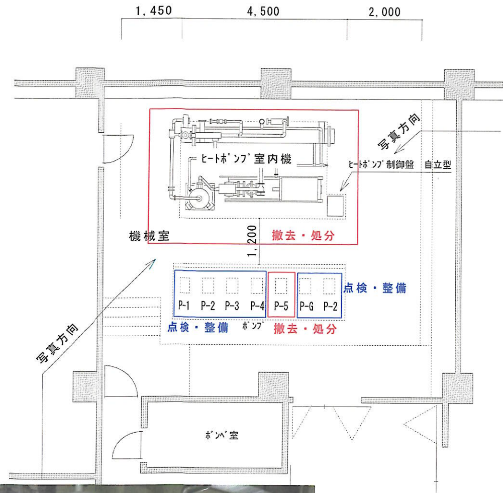
機械室概略平面図 S=1:100
