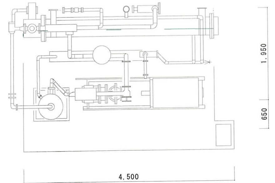
ヒートポンプ室内機正面図 S=1:50
