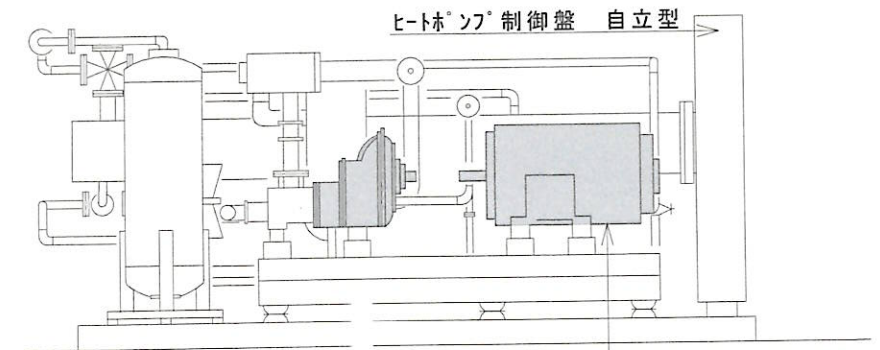
ヒートポンプ室内機正面図 S=1:50
